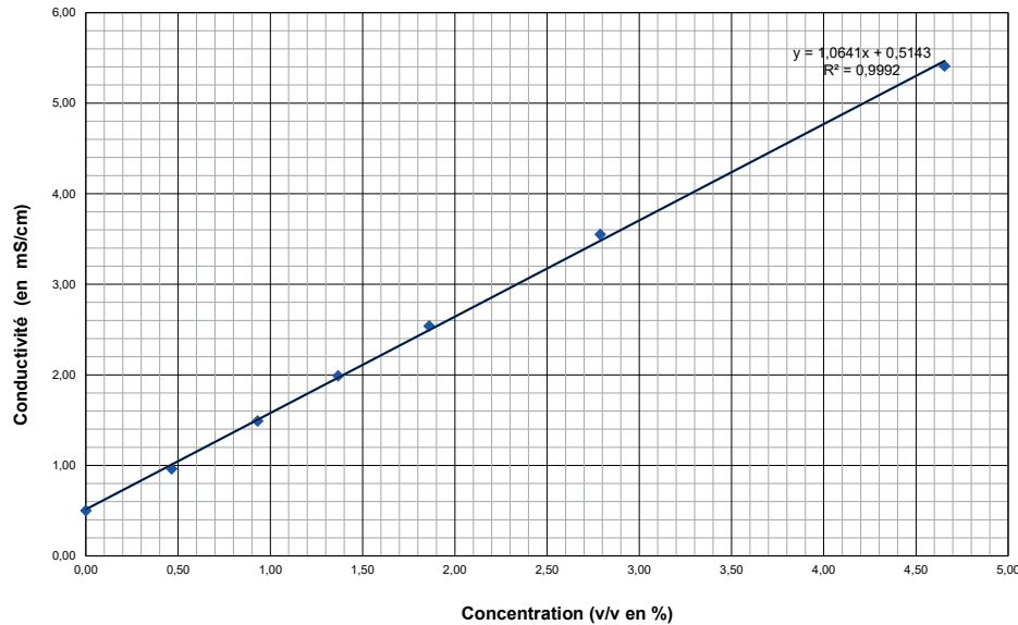
Courbe de conductivité à 25°C du $FA710 - DETERQUAT DDM NF - V1 Courbe réalisée avec une eau de dureté = 19°f avec le conductimètre WTW Cond 3310
